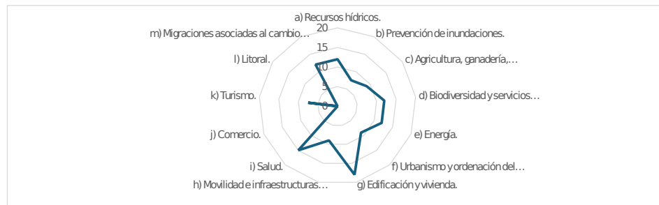
Figura 47. Diagrama resumen de las valoraciones del riesgo del impacto "cambios en la frecuencia, intensidad y magnitud de los incendios forestales" en las áreas estratégicas seleccionadas en El Viso del Alcor. Fuente: Elaboración propia
