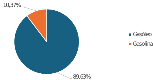
Figura 30. Distribución del consumo de combustibles en automoción en 2021.
