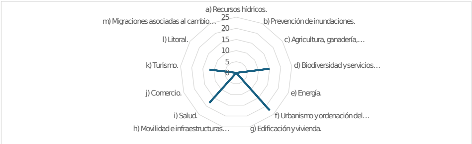
Figura 48. Diagrama resumen de las valoraciones del riesgo del impacto "pérdida de calidad del aire" en las áreas estratégicas seleccionadas en El Viso del Alcor. Fuente: Elaboración propia
