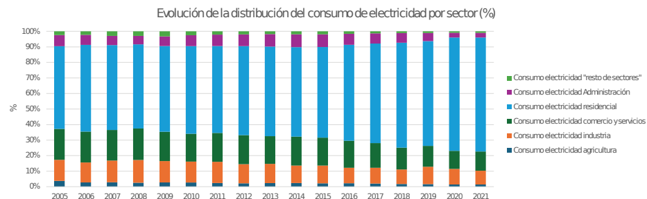
Figura 23. Evolución de la distribución del consumo de electricidad por sector de 2005 a 2021. Fuente: Elaboración propia a partir de datos procedentes de la aplicación HCM de la Junta de Andalucía
