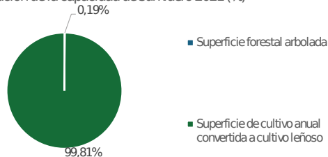
Figura 18. Distribución de la capacidad de sumidero en 2021 por actividad. Fuente: Elaboración propia a partir de datos procedentes de la aplicación HCM de la Junta de Andalucía
