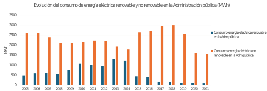
Figura 24. Evolución del consumo de electricidad en la Administración pública desglosados por su origen, renovable y no renovable, de 2005 a 2021. Fuente: Elaboración propia a partir de datos procedentes de la aplicación HCM de la Junta de Andalucía
