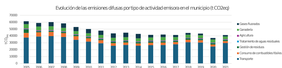
Figura 5. Evolución de las emisiones difusas de 2005 a 2021 desglosadas por tipo de actividad. Fuente: Elaboración propia a partir de datos procedentes de la aplicación HCM de la Junta de Andalucía
