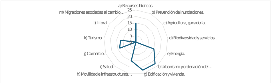
Figura 56. Diagrama resumen de las valoraciones del riesgo del impacto "modificaciones en el sistema eléctrico: generación, transporte, distribución, comercialización, adquisición y utilización de la energía eléctrica" en las áreas estratégicas seleccionadas en El Viso del Alcor.
