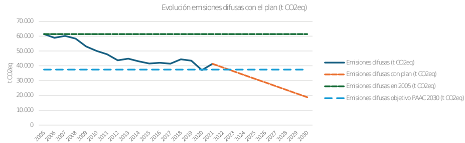
Figura 61. Evolución de emisiones difusas esperadas en El Viso del Alcor con la aplicación del PMCC. Fuente: Elaboración propia
