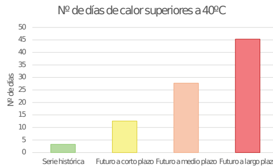
Figura 39. Diagrama de variación del número de días en los que se superan los 40 °C al año en El Viso del Alcor para la serie histórica de 1961 a 1990 y para los horizontes temporales de futuro a corto, medio y largo plazo.
