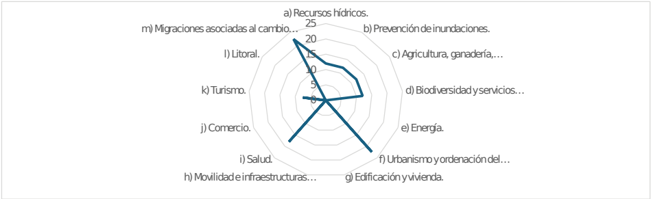
Figura 46. Diagrama resumen de las valoraciones del riesgo del impacto "pérdida de biodiversidad y alteración del patrimonio natural o de los servicios ecosistémicos" en las áreas estratégicas seleccionadas en El Viso del Alcor. Fuente: Elaboración propia
