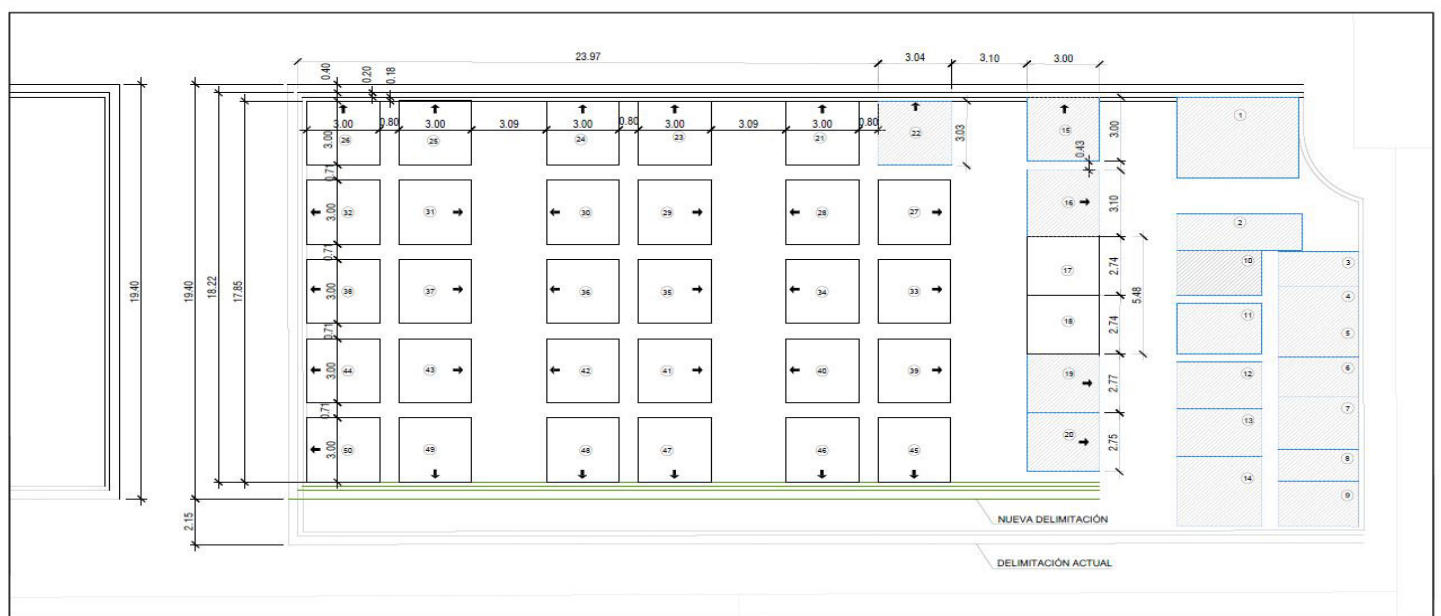
DISTRIBUCIÓN Escala 1: 150
